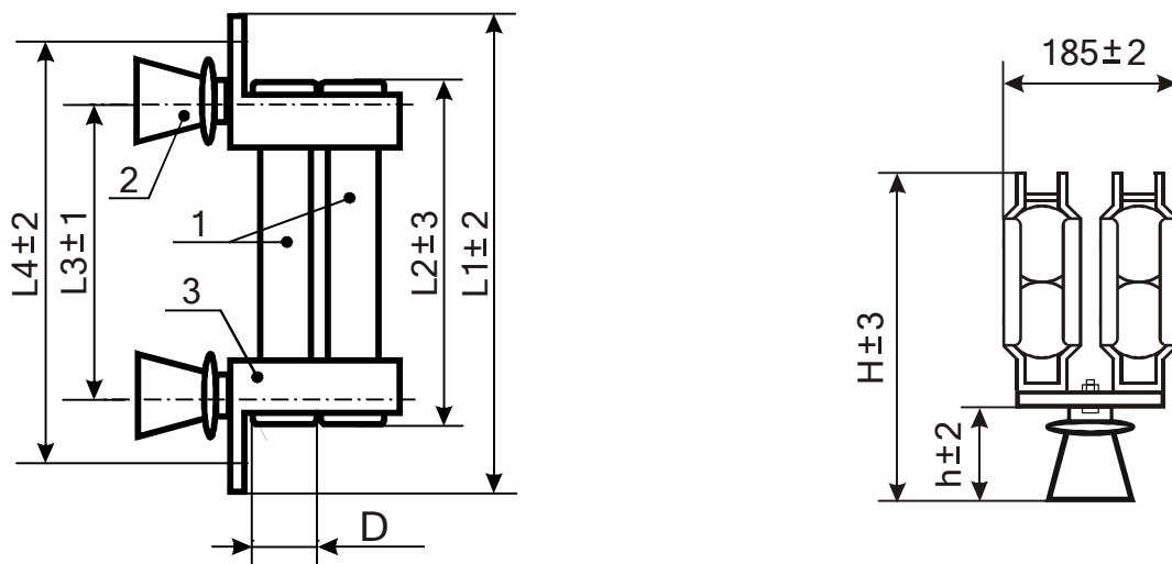
1 – патрон; 2 – ізолятор; 3 – контакт. Мал. 7.
