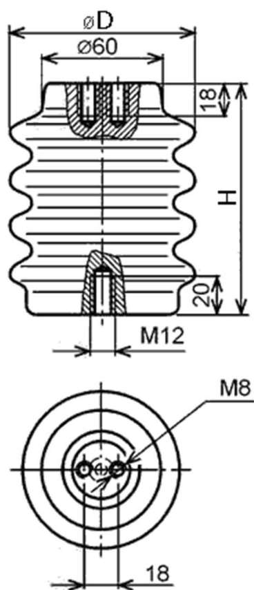
Изолятор ИОР
